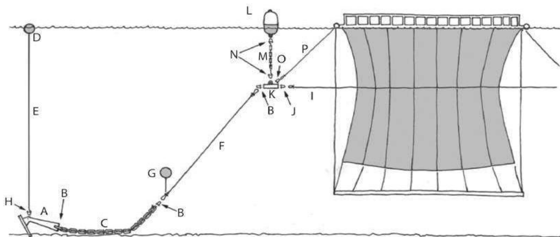
Hình 7. Hệ thống neo
